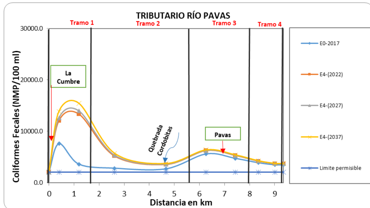
Figura 29 Resultados del Escenario 4 para los coliformes fecales (patógenos) en el río Pavas
