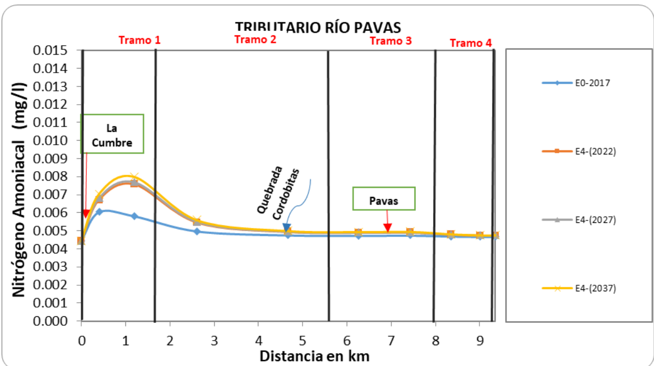
Figura 27 Resultados del Escenario 4 para el nitrógeno amoniacal en el río Pavas
