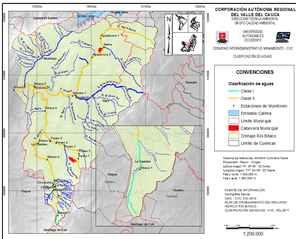
Figura 37 Clasificación de las aguas de los ríos Bitaco, Pavas y el sistema quebrada Aguamona-río Grande
